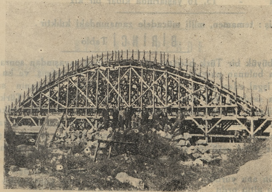
— Memleketimizde Bayındırlık varlıklarından — Kızılrnak köprüsü inşaatı ilerliyor
